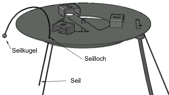
Seilhalter
